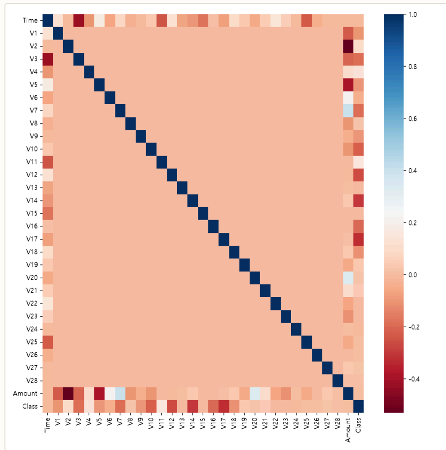
그림 3-3. 31개 변수 전체의 피어슨 상관관계 히트맵(card_df.corr(), cmap='RdBu'). 파란색이 양의 상관, 빨간색이 음의 상관이다. V1~V28 블록이 대각선만 진하고 나머지는 균일한 것은 PCA 축들이 서로 직교하기 때문이며(§3.1.3), 실제로 V1~V28 사이의 상관관계 최댓값은 |r|=0.0000 이다. 색이 뚜렷하게 갈리는 곳은 맨 위 Time 행, 아래 Amount 행, 맨 아래 Class 행뿐이다.
