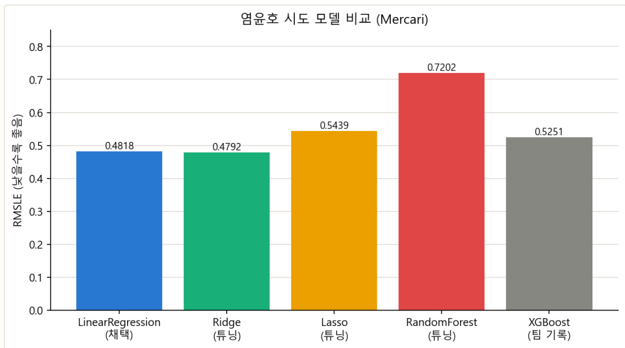
그림 5-5. 모델 비교. XGBoost는 팀 공유 기록(40만 행 서버샘플) 기준.
